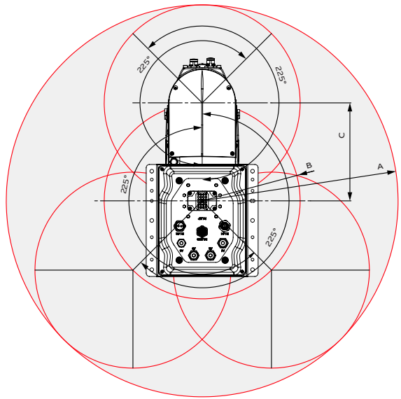
IRB 910INV-3/0.35 和 IRB 910INV-6/0.55, 工作范围图例
