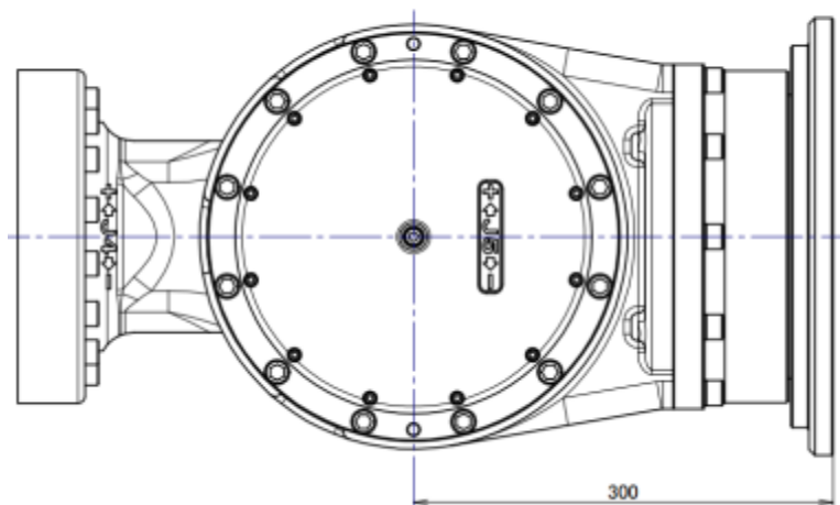
标准法兰
