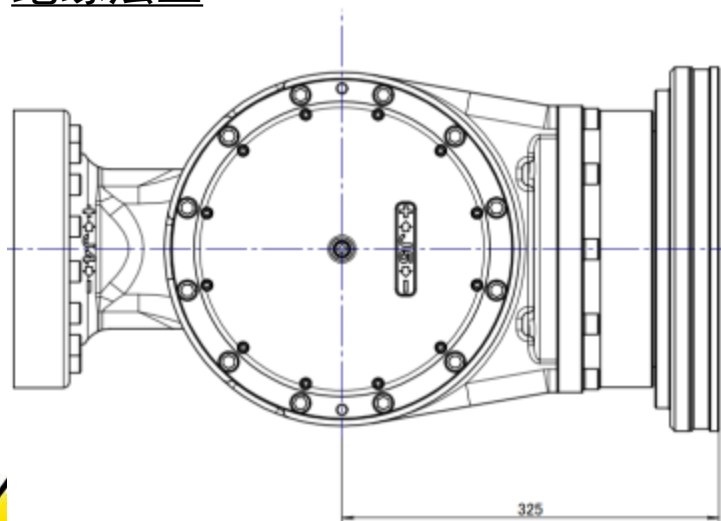
绝缘法兰
