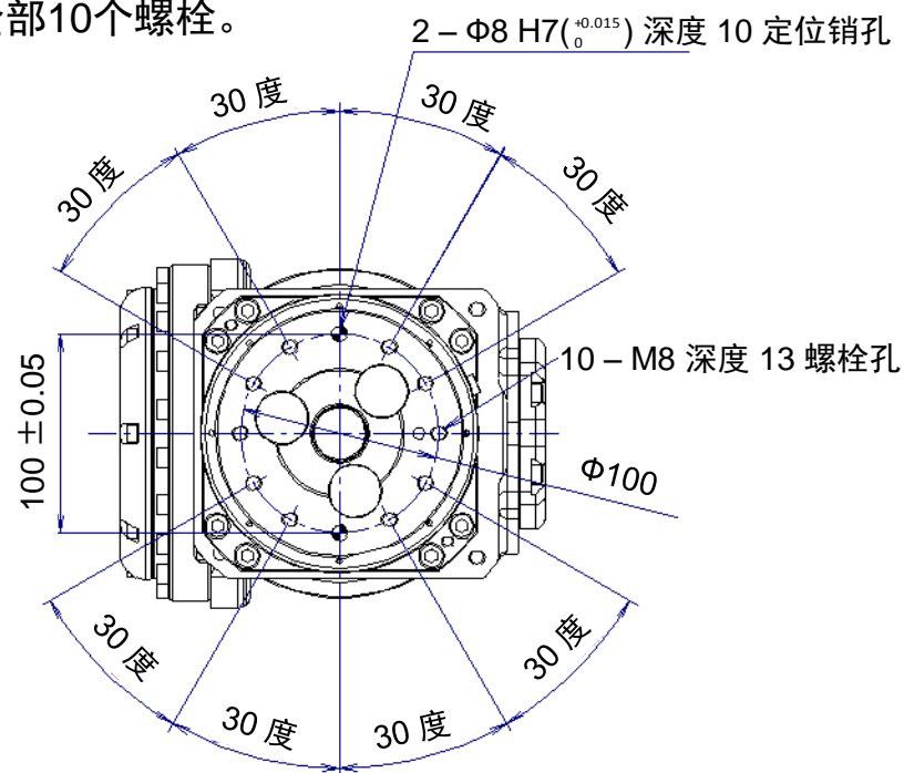
ISO 法兰
