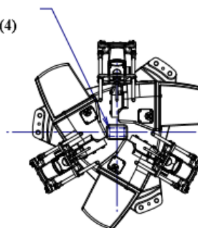
剖面 C-C
