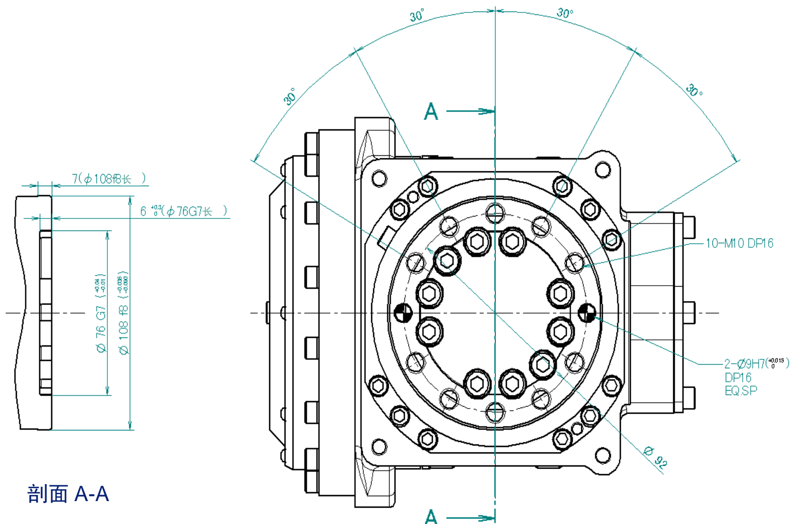
特殊法兰盘
