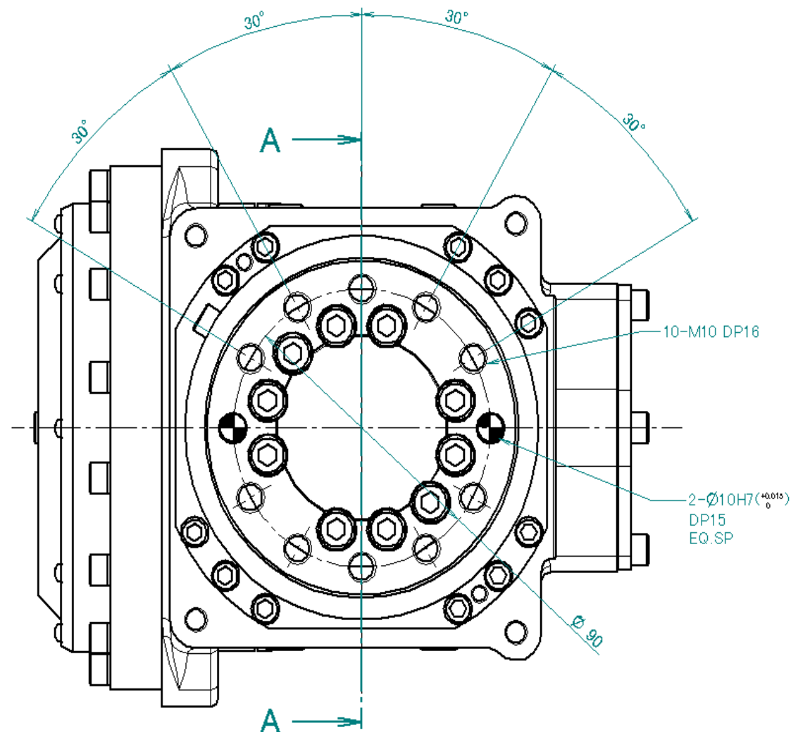
FANUC 法兰盘
