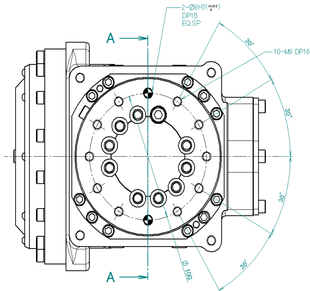
ISO 法兰盘
