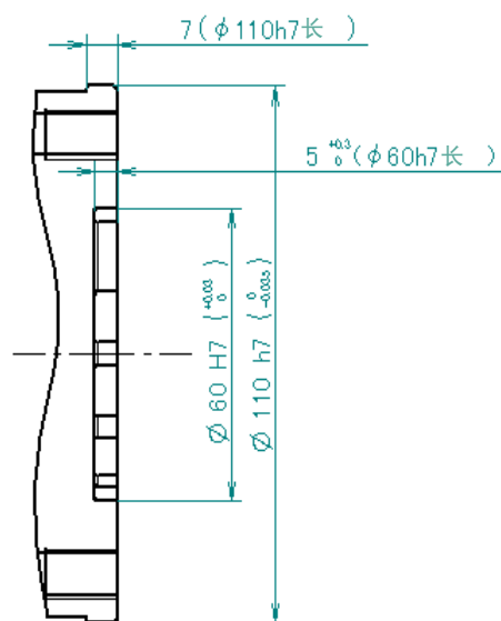
剖面 A-A
