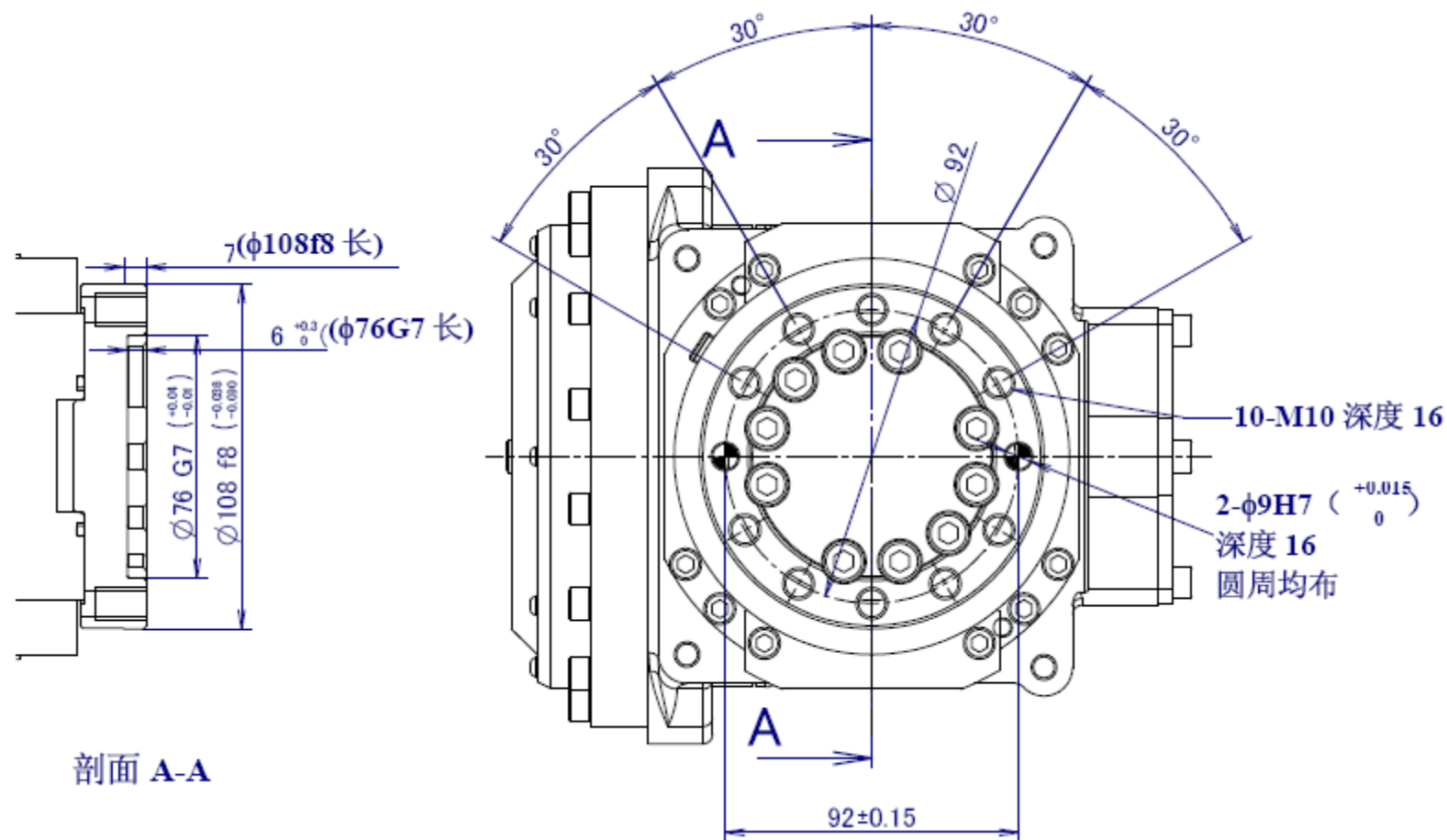
特殊法兰盘
