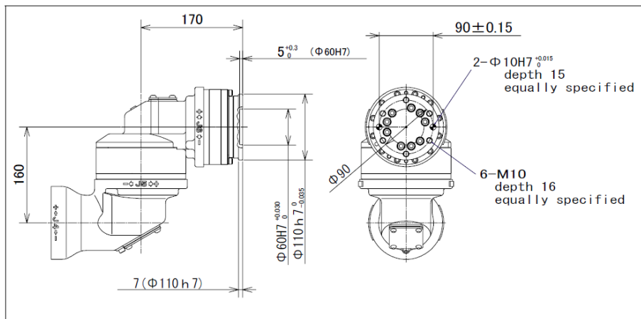
Fig.2.4 (d) End effector mounting face (Offset wrist, Standard flange)
