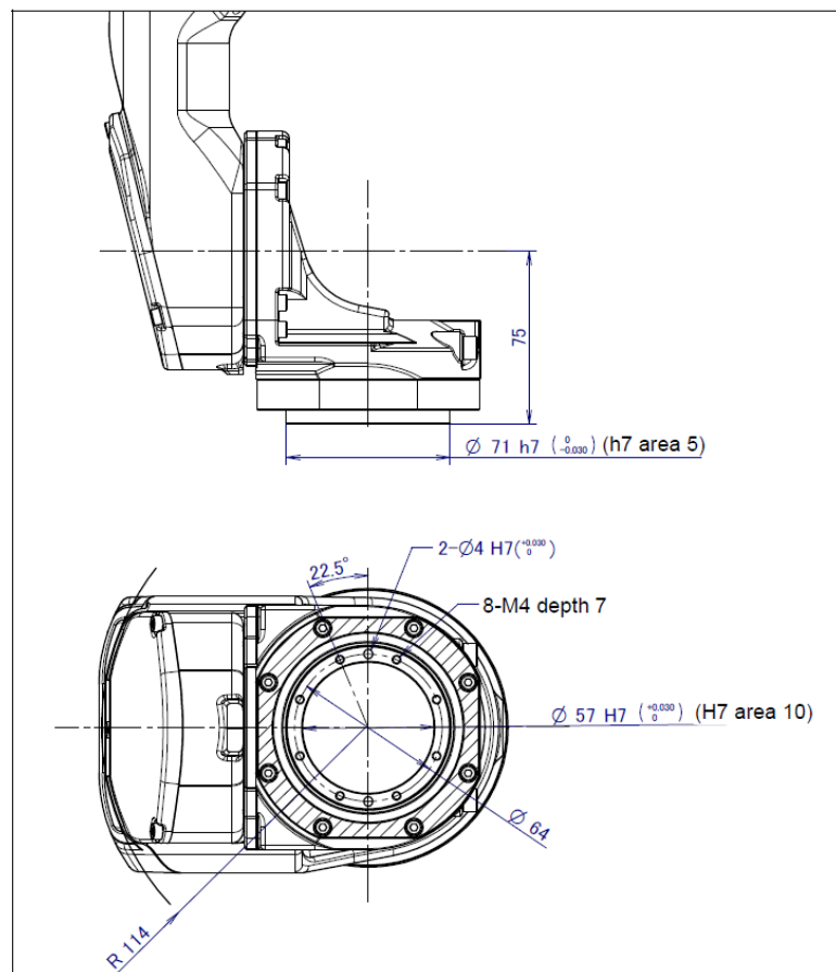
M-10iD/8L
